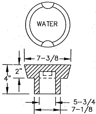
VALVE BOX DROP LID
